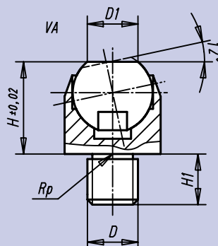
Forme C A embout fileté, bille avec plat rectifié
