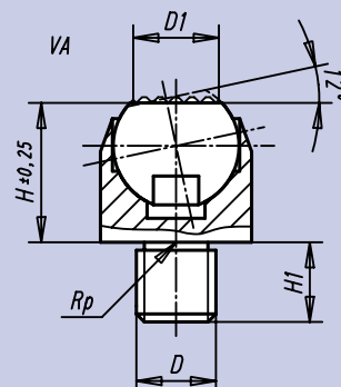
Forme F A embout fileté, bille avec picots
